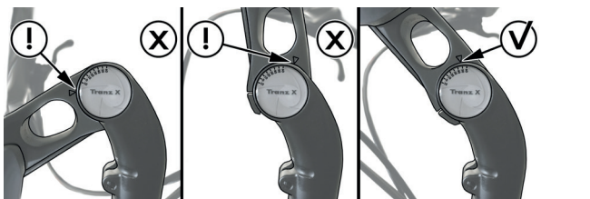
Abbildung 11: Bleiben Sie innerhalb des Bereichs, der auf der Seite des Vorbaus angeben ist.
