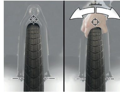
Afbeelding 36: Speling in de achternaafas controleren
