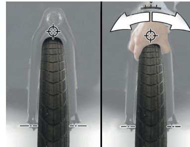
Abbildung 36: Überprüfung des Spiels der hinteren Nabenachse
