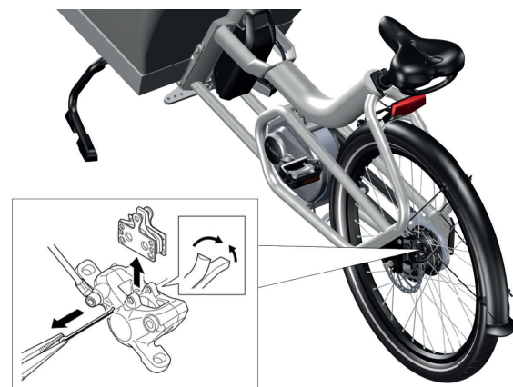
Image 39 : Retrait des plaquettes de frein afin de vérifier leur état d'usure
