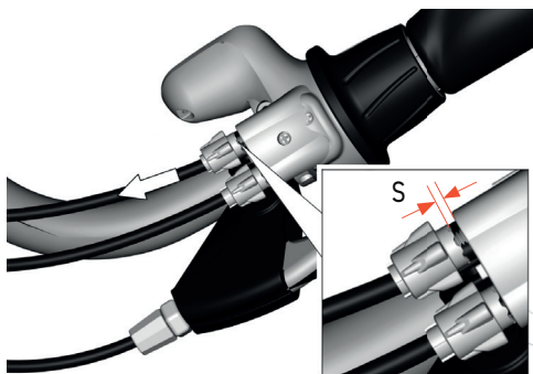
Afbeelding 40: Kabelspeling controleren
