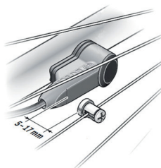
Abbildung 31: Abstand zwischen dem Geschwindigkeitssensor und dem Geschwindigkeitssensormagneten
