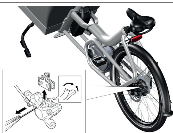
Abbildung 39: Entfernen der Bremsbeläge, um sie auf Verschleiß zu prüfen
