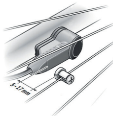
Image 31 : Distance entre le capteur de vitesse et l'aimant de rayon du capteur de vitesse
