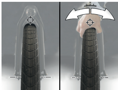
Image 36 : Vérifier le jeu sur l'axe du moyeu arrière
