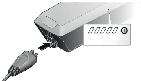
Abbildung 29: Ladegerätstecker in die Ladebuchse am Akku stecken.
